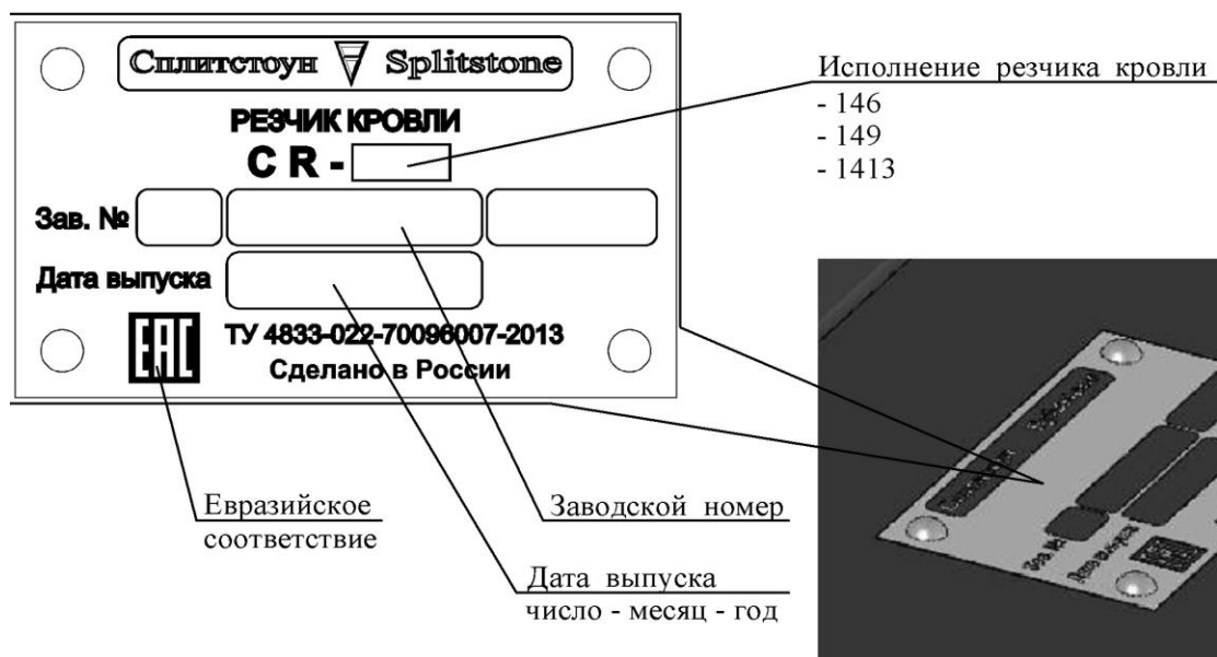
Рисунок 2 – Маркировка
