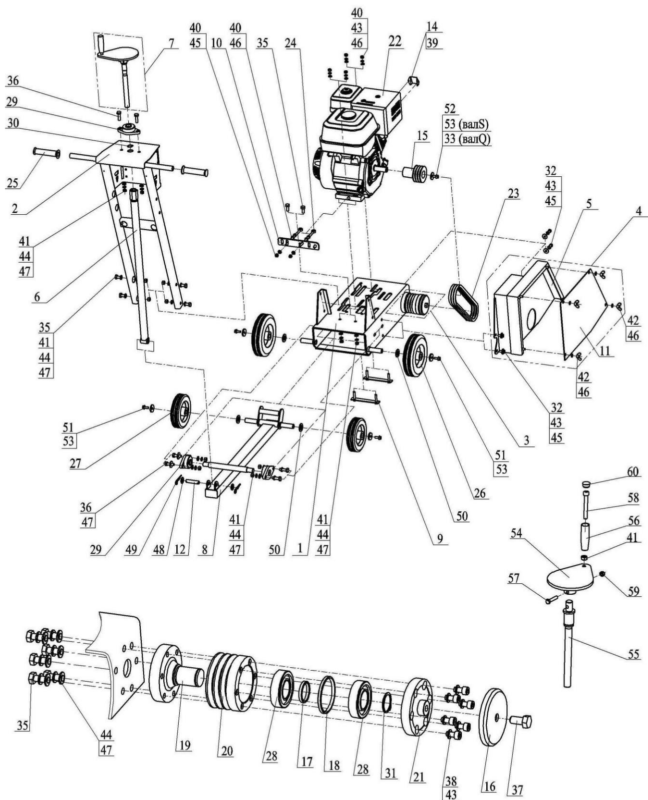
Рисунок 10 – Компоновка резчиков
